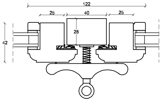
Vandret snit i 2 fags sidehængt forsatsramme
